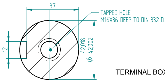
Przekrój A-A 1:1
